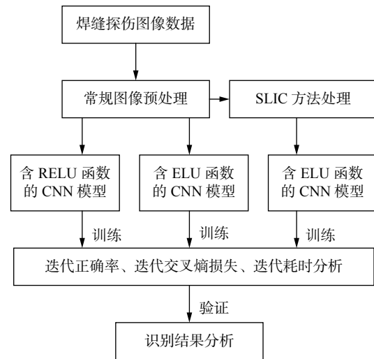
图 3 缺陷识别流程图
